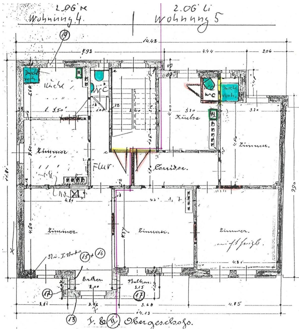
Grundriss 2. Obergeschoss
